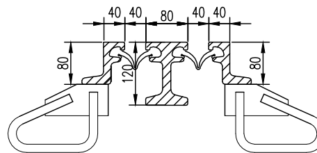
锚筋组处断面图
