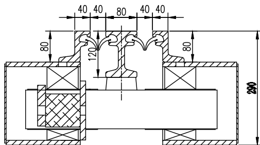
位移箱处断面图
