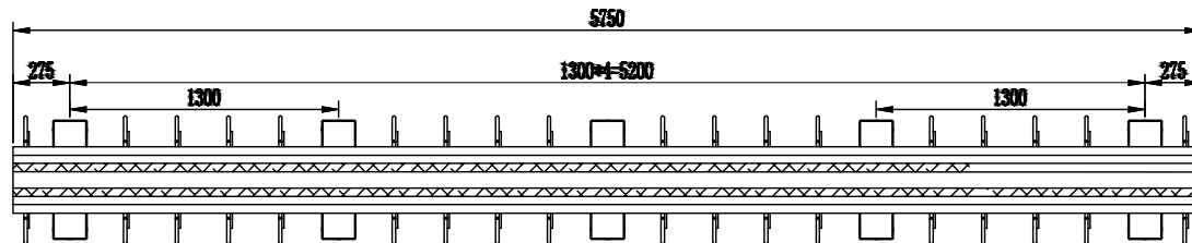
平面布置图
