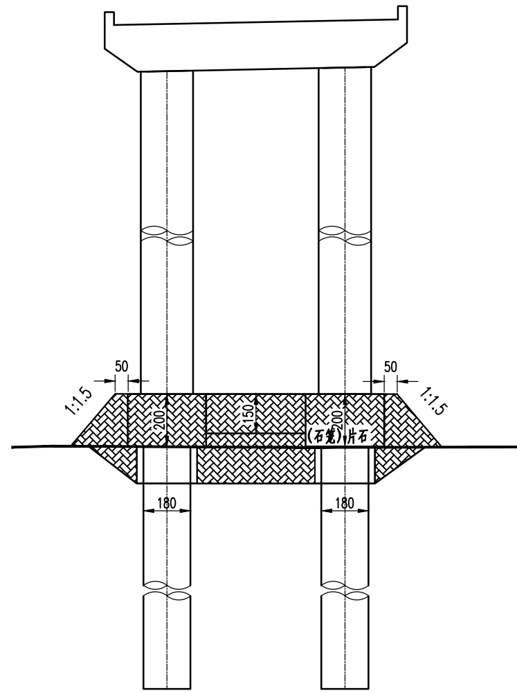
立面示意图
