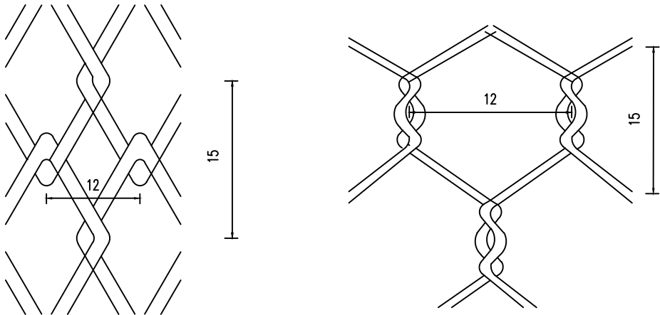
钢丝网大样图
