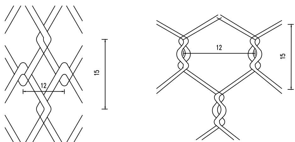
钢丝网大样图
