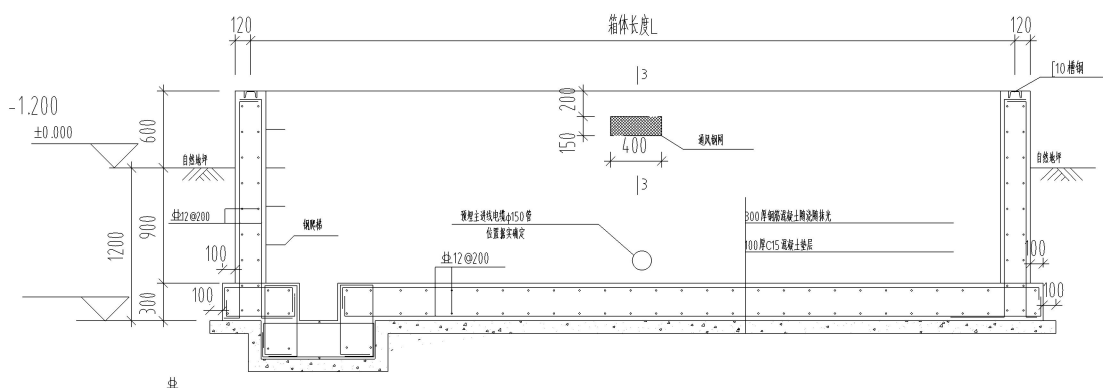
1-1剖面图
