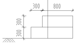
台阶做法
