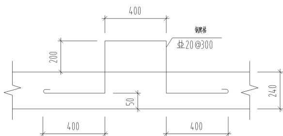
钢爬梯详图
